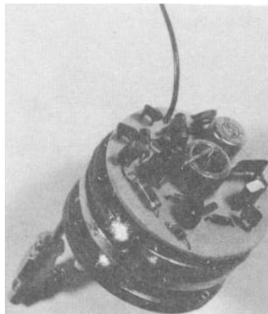
Fig. 10 - L-Band Transmitter
