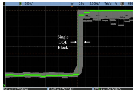
B) DQM Step Response
